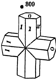
Staurolite.
